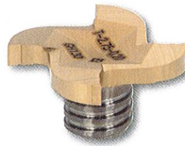
VST***-4/6 溝加工用 4, 6 枚刃 溝幅：0.76 - 10 mm
